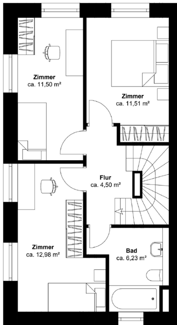
1. Obergeschoss
